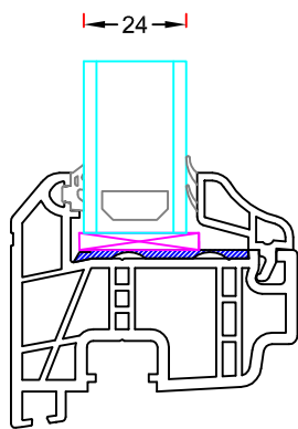
24mm glas 22,5mm keulet glasliste med grå bånd.
