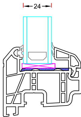
24mm glas 22,5mm glasliste med grå bånd.
