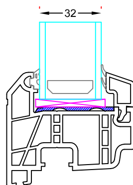
32mm glas 14,5mm glasliste med grå bånd.
