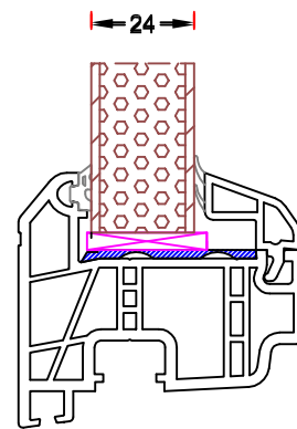
24mm fyldning 22,5mm glasliste med grå bånd.
