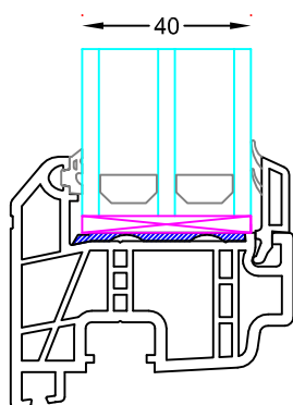
40mm glas 6,5mm glasliste med grå bånd.
