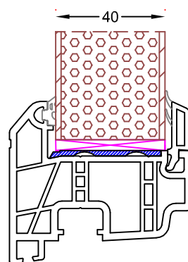
40mm fyldning 6,5mm glasliste med grå bånd.
