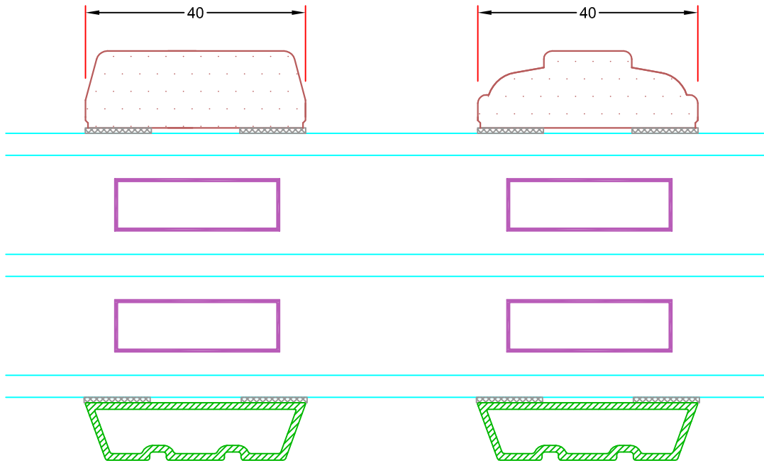
40mm energisrosser med og uden kehlung. Kehling kun til indvendig
